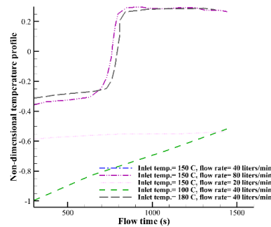
(d) 10 mm above heat transfer fluid tube
